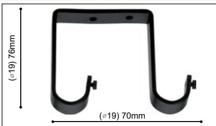
SopORTE Techo Doble
