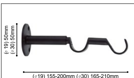
SopORTE Pared Doble Redondo Extensible
