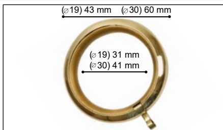
Anillas con teflón Rings with teflon / Anneaux avec teflon
